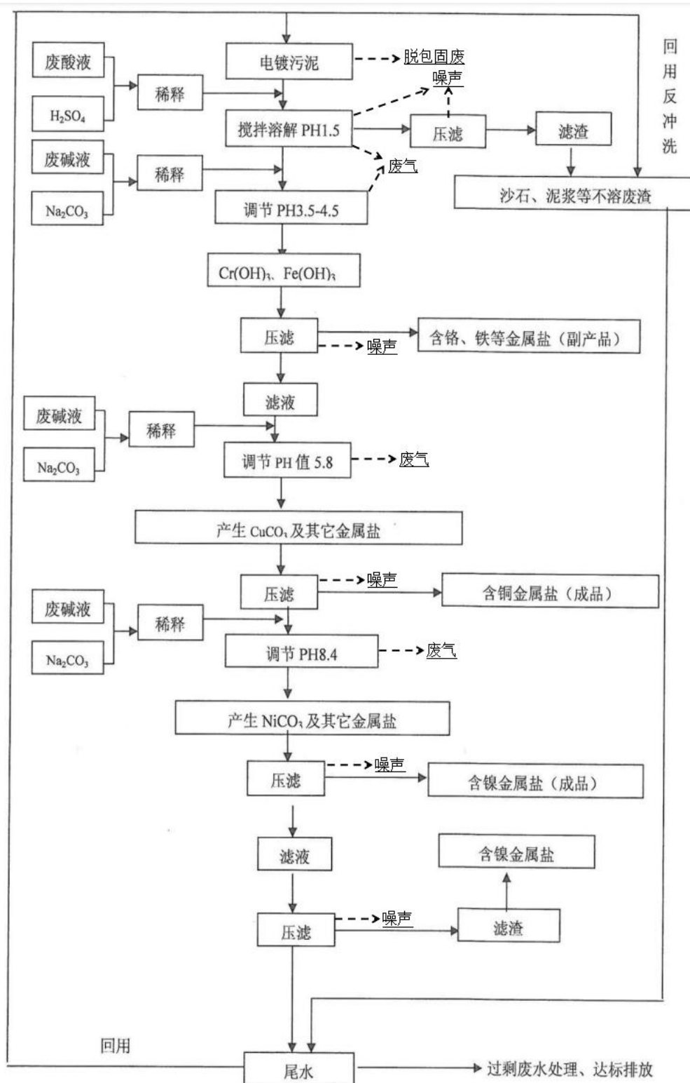
图 4.1-3 综合污泥回收利用工艺流程图
