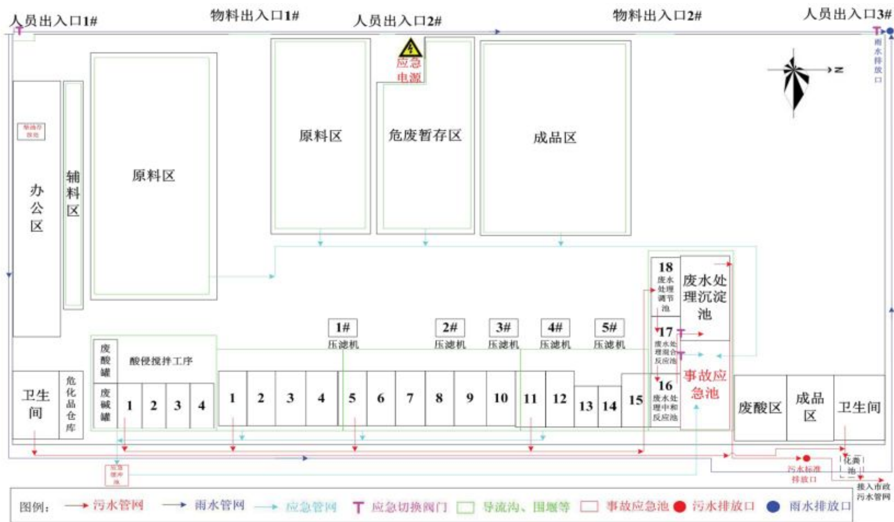
图 4.2-2 宜境公司雨污管道布置示意图
