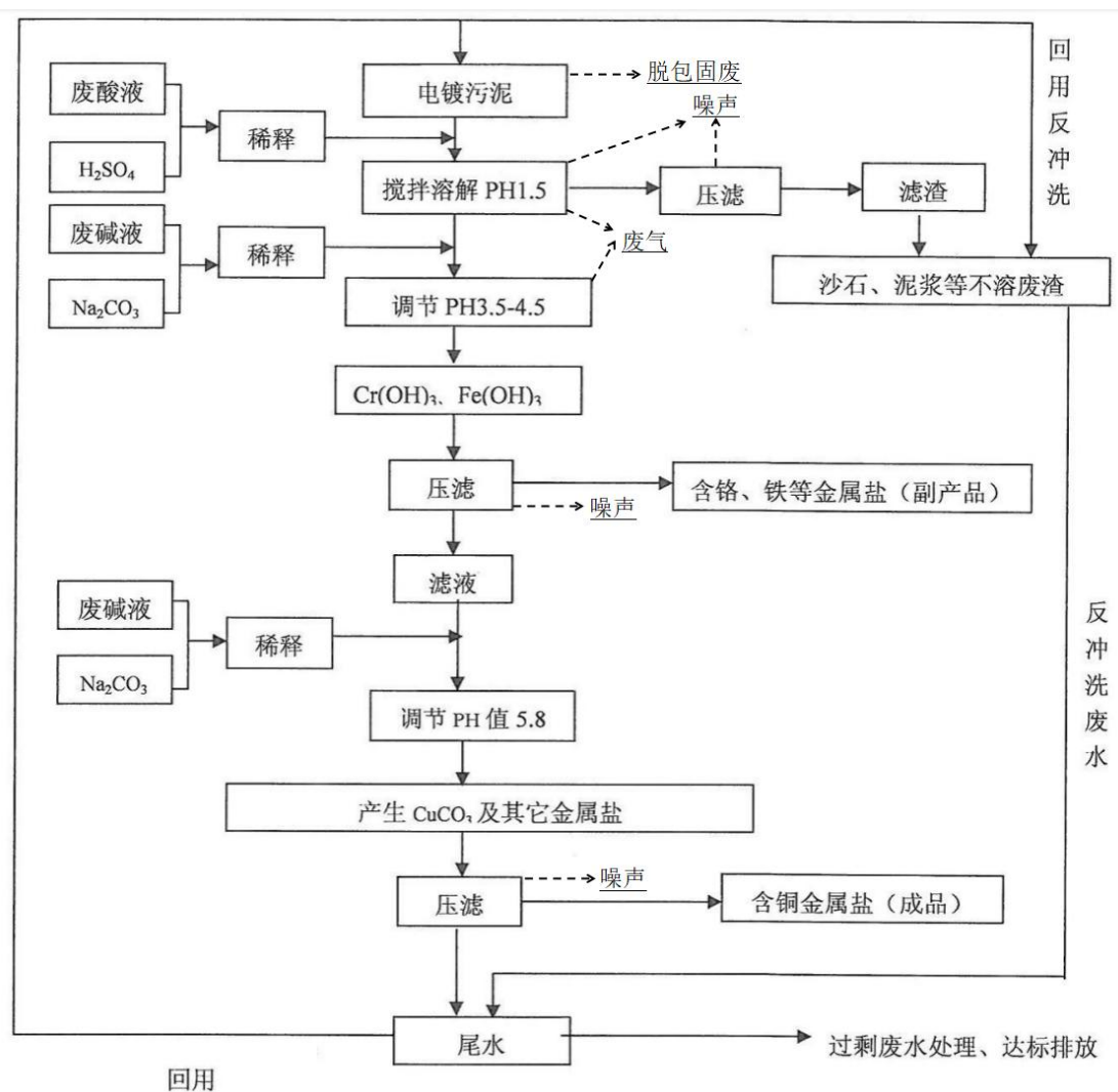
图 4.1-1 含铜污泥回收利用工艺流程图
