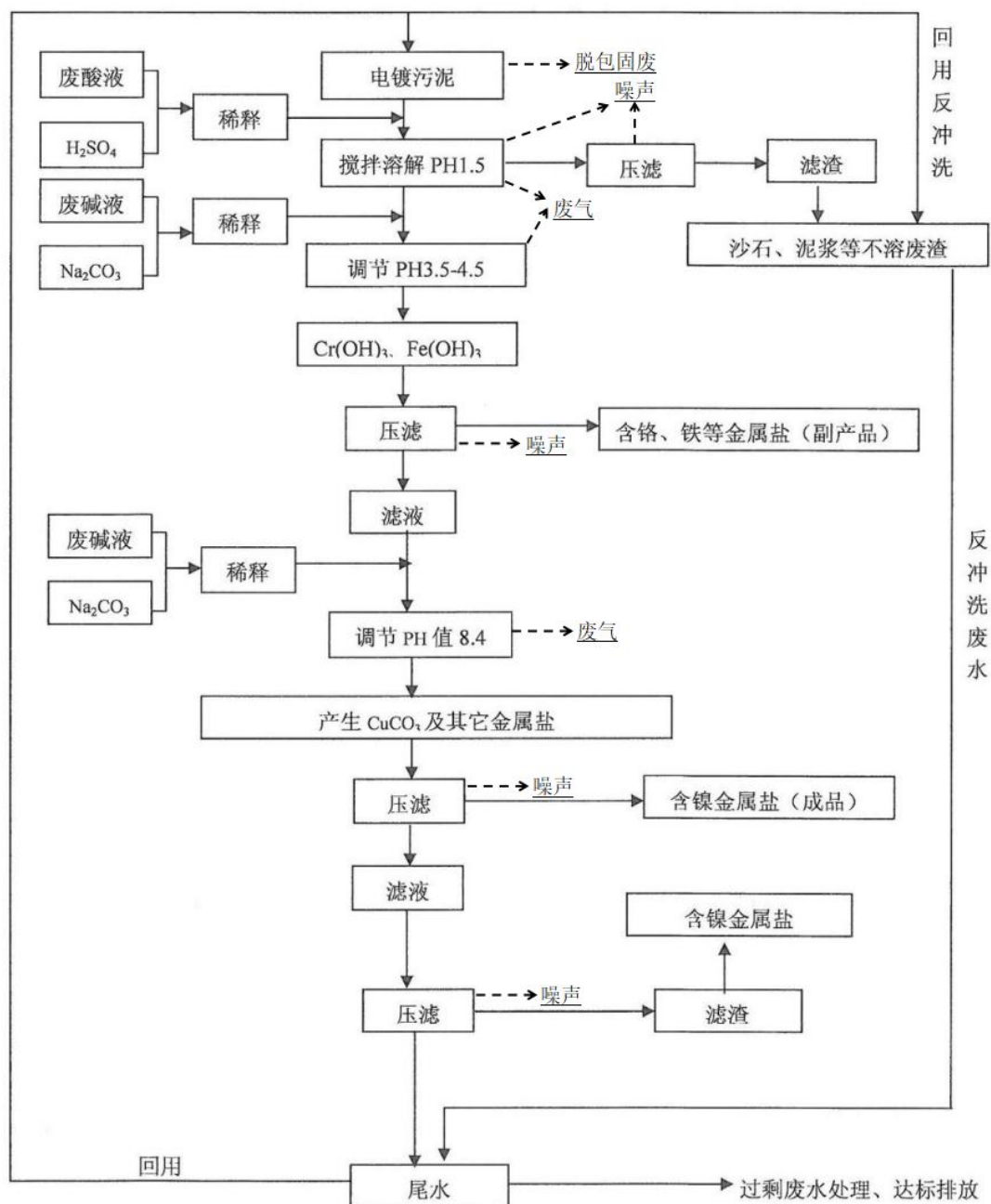
图 4.1-2 含镍污泥回收利用工艺流程图
