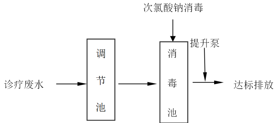
图 4 项目污水处理工艺流程图
