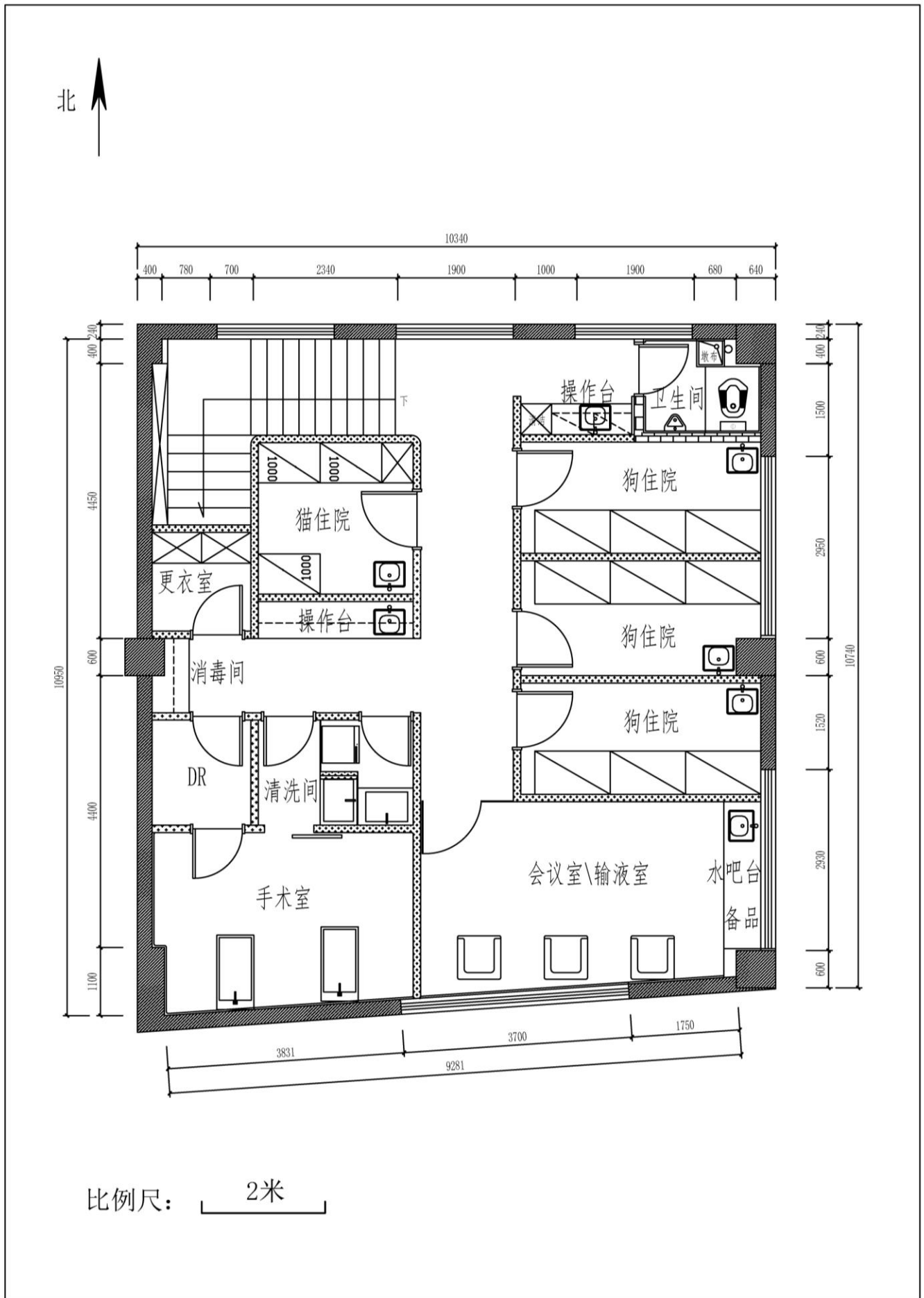
附图 4 建设项目二层平面布置图
