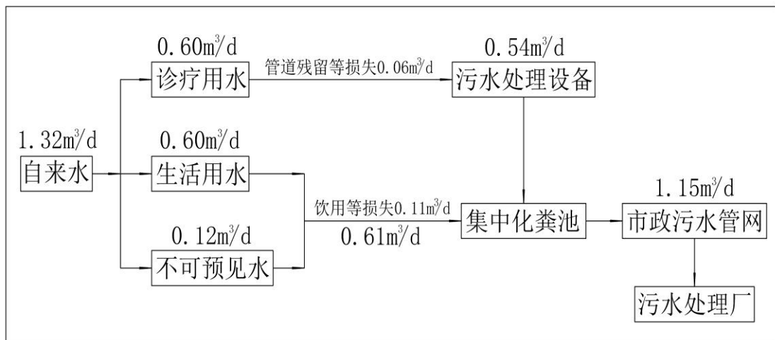
图 3 项目水平衡图
