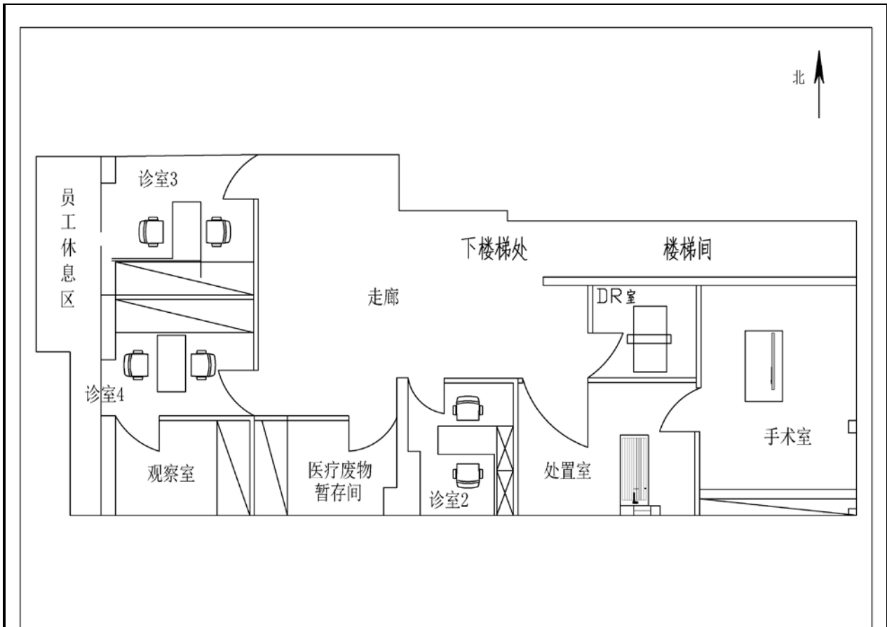
图4 项目二层平面布置图（1:100）
