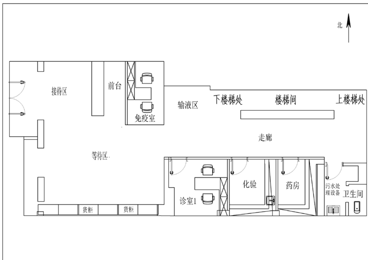
图3 项目一层平面布置图（1:100）
