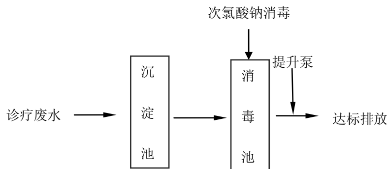
图 5 项目污水处理工艺流程图
