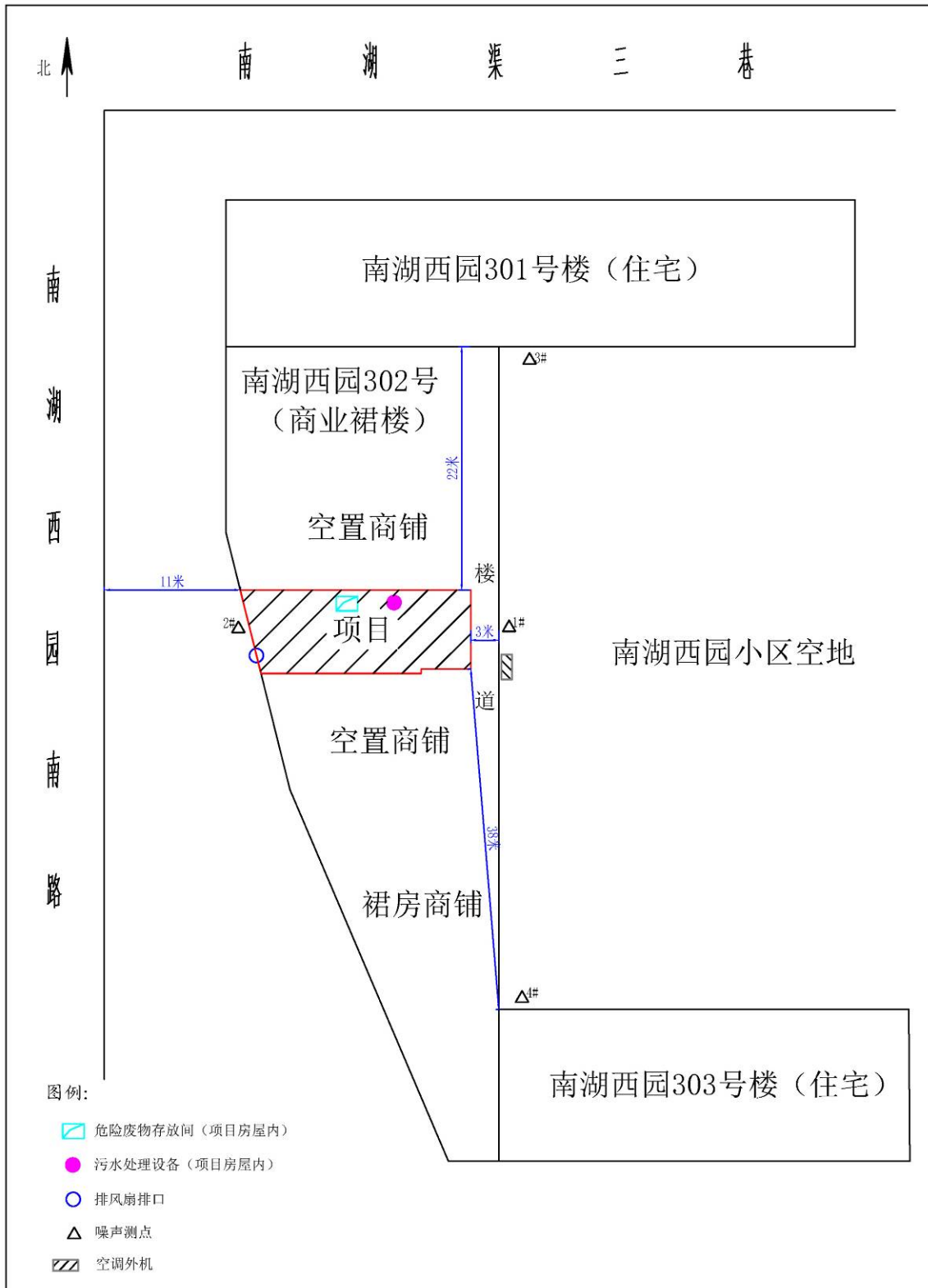
图2 项目周边关系图（1:500）
