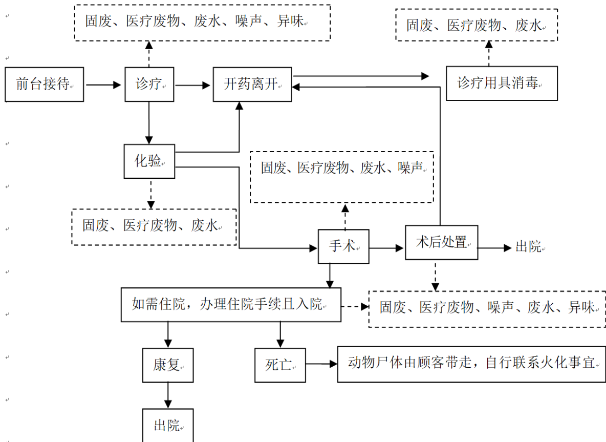
图 4 项目运营期工艺流程和产污环节示意图
