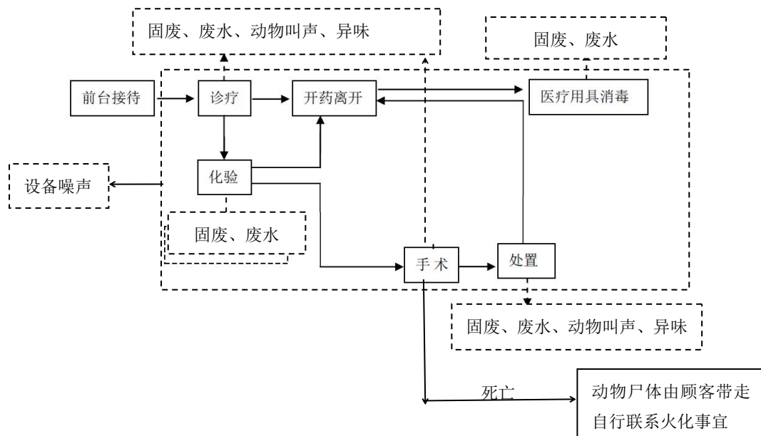
运营期工艺流程及产污环节
