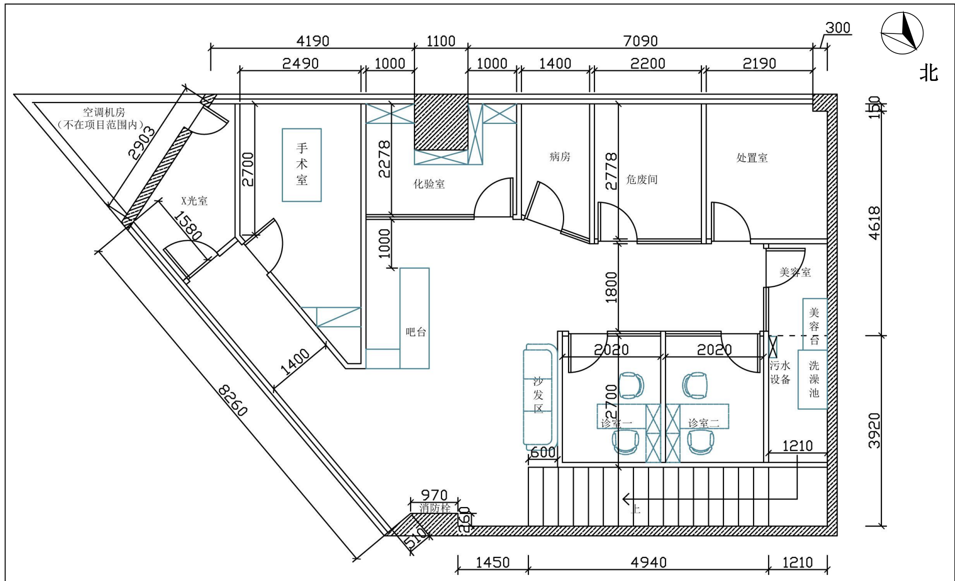
图3 建设项目平面布置图
