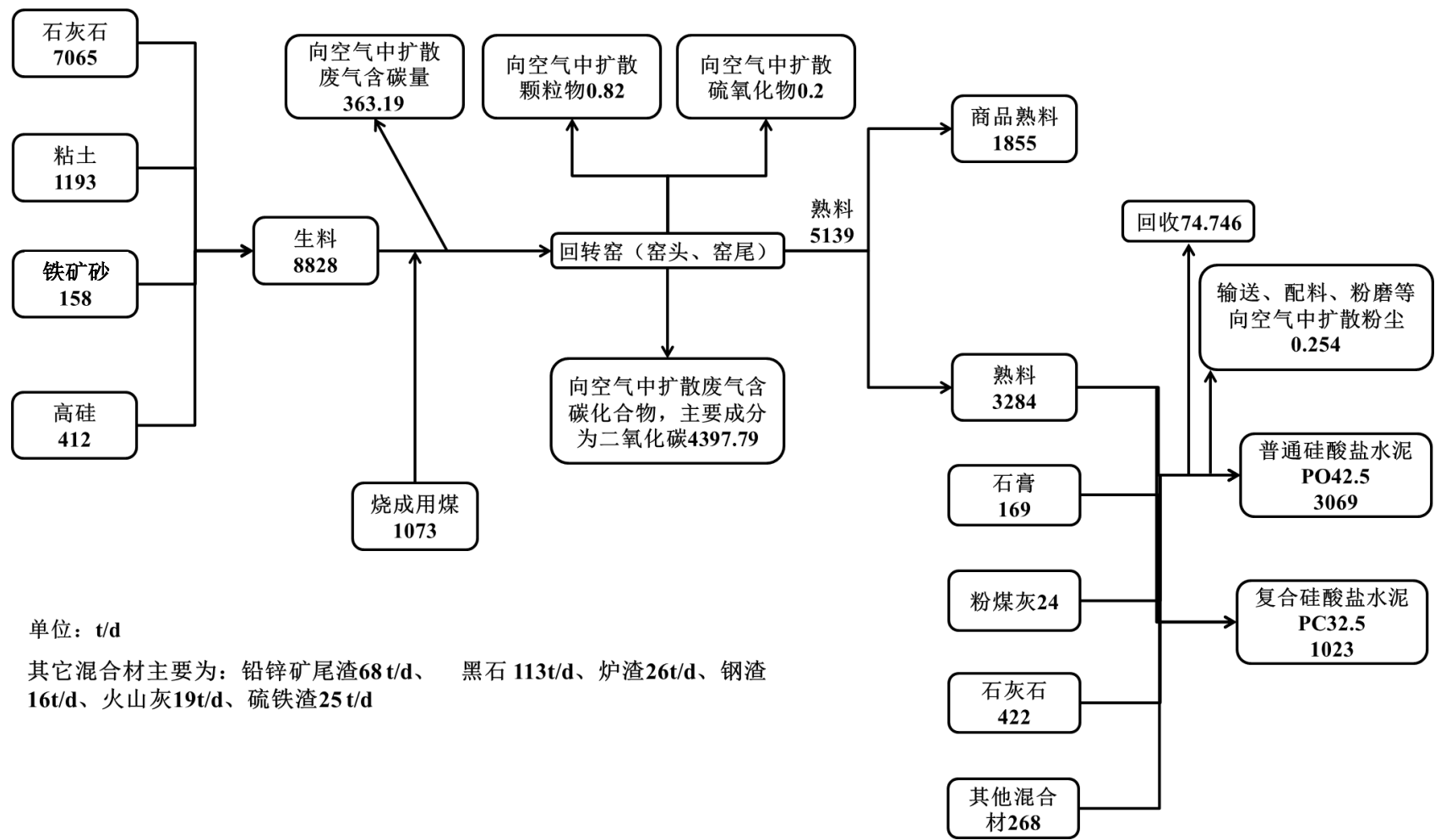
图 3.3-1 项目物料平衡图
