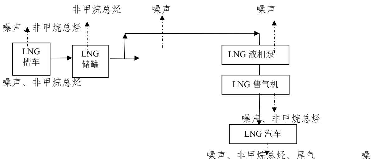
图 3 LNG 加气站工艺流程与产污节点图
